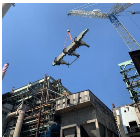
Desmuntatge bigues guirder estructura principal
